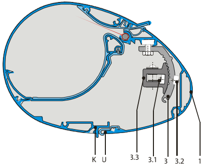
Abbildung 2 (Systemdarstellung)
