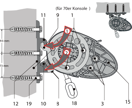
Abbildung 2 (Systemdarstellung)
