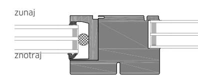
ALWOOD v kombinaciji s SISTEMOM LOFT.
