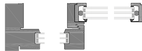
Dvižno-drsna vrata les-aluminij z zasteklitvijo brez vidnih okvirjev.
